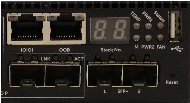
Abbildung 1-15. N30xx Nahaufnahme
