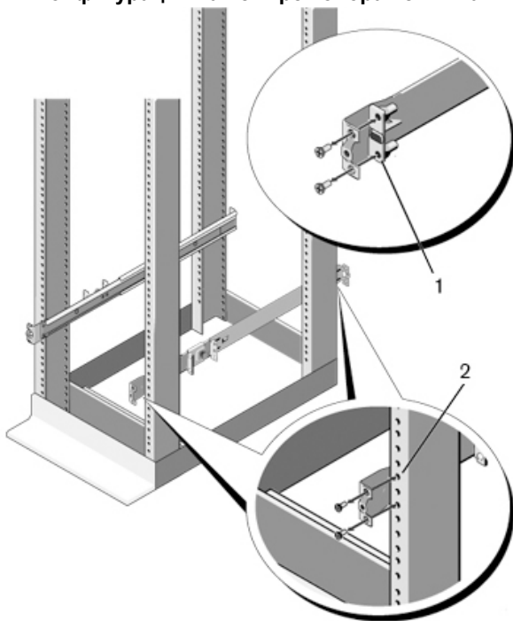
Рисунок 1-22. Конфигурация на четырех опорах с винтами
