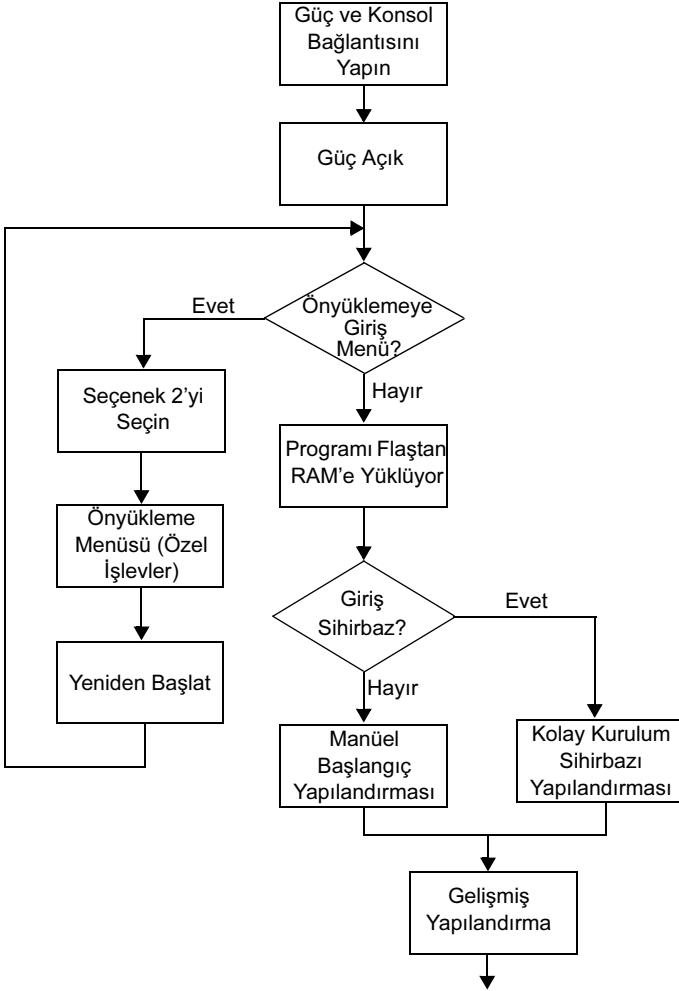
Şekil 1-9. Kurulum ve Yapılandırma Akış Çizelgesi
