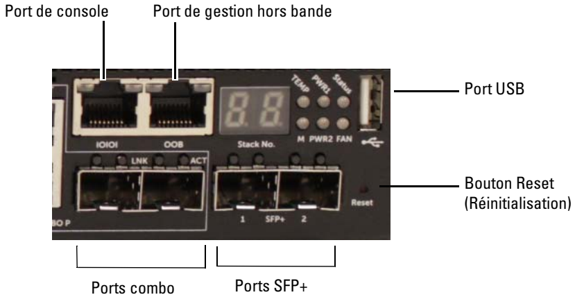
Figure 1-14. Ports supplémentaires présents sur les commutateurs N30xx
