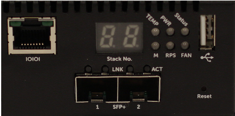
Abbildung 1-2. N2024 Nahaufnahme
